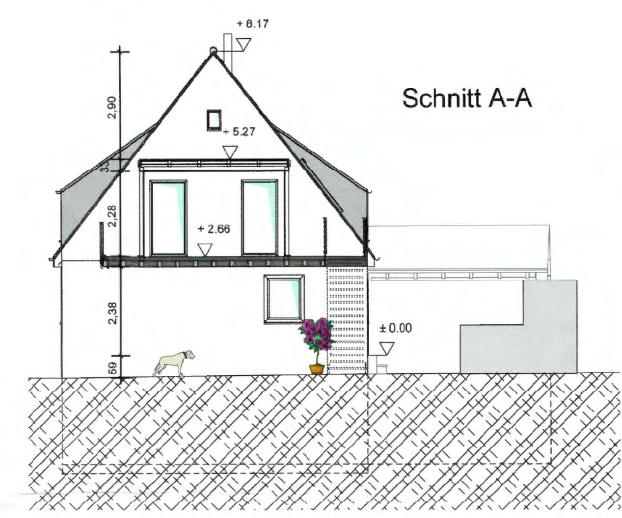
Anbau eines Balkones mit Wintergarten an ein bestehendes Wohnhaus
